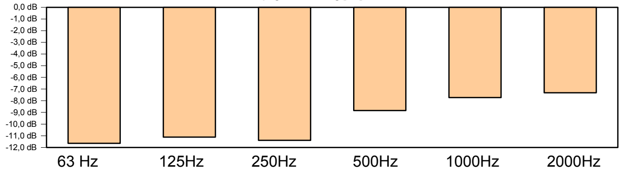
Schallpegelminderung [dB]
